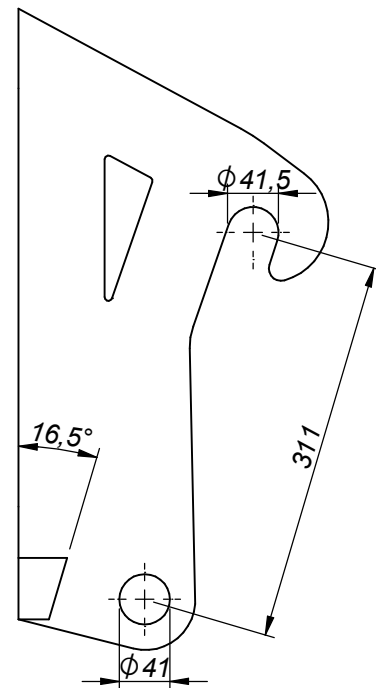
PRZEKRÓJ A-A
